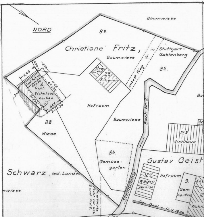
Plan oben von 1956, er wurde gefertigt am 26. April desselben Jahres. Das Baugesuch betraf den Abbruch und Wiederaufbau des Gebäudes über dem Kellergeschoß. Architekt war Jacob Bauer, Öhringen
